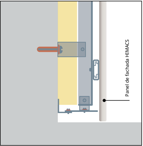
Tapajuntas de base (tapajuntas inferior)
