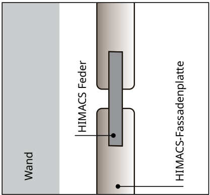
Nut- und Feder-Verbindung (mit Feder-Element aus HIMACS)
