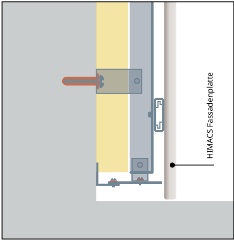
Sockel-Abschluss (unterer Abschluss)
