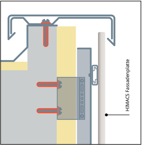
Attika-Abschluss (oberer Abschluss)
